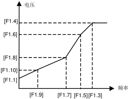
图 6-6 V/F 自定义曲线设定
