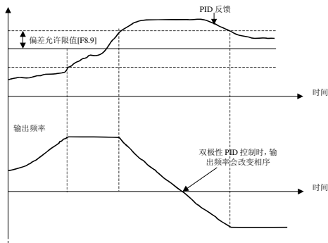
图 6-30 双极性 PID 控制方式
