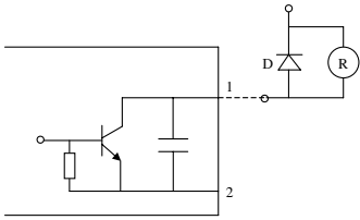
图 6-12 OC 输出端子的内部线路
