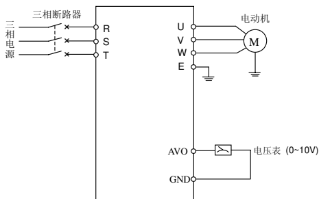
图 9-1 基本接线图
