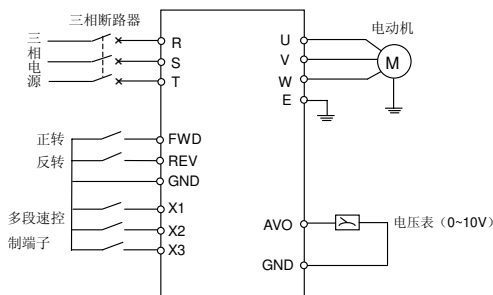
图 9-2 基本接线图
