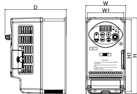
图 2-2-B 变频器安装尺寸 II
