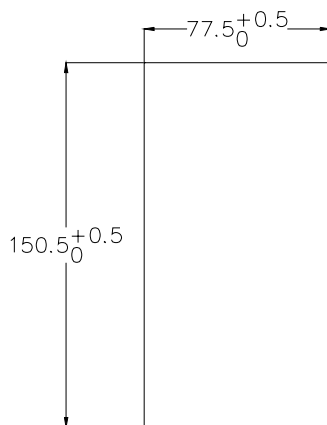
图-B 操作面板底座安装开孔尺寸
