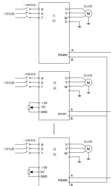
图 9-4 基本接线图
