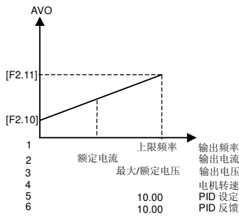
图 6-11 模拟输出端子的模拟输出内容
