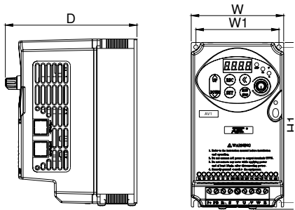
图 2-2-A 变频器安装尺寸 I
