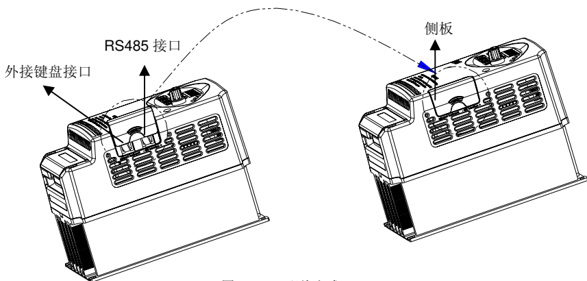
图 3-4-B 配线方式 II
