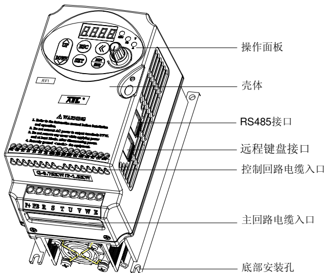
图 1-1 I 类变频器部件名称
