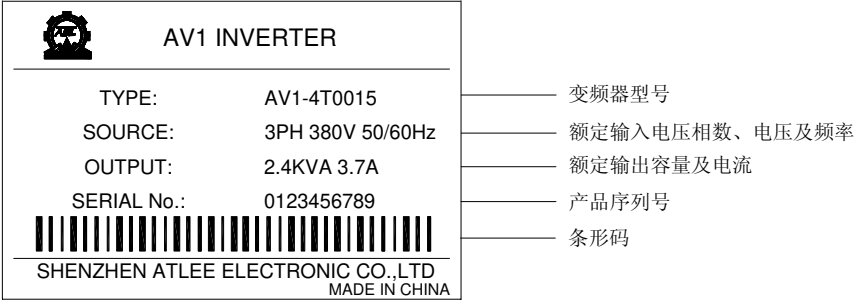
图 1 变频器铭牌数据
