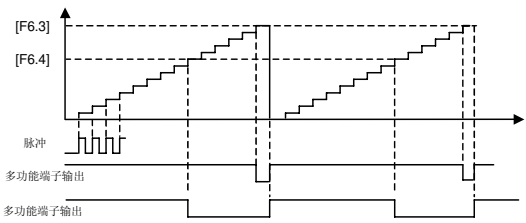
图 6-25 内部计数器功能
