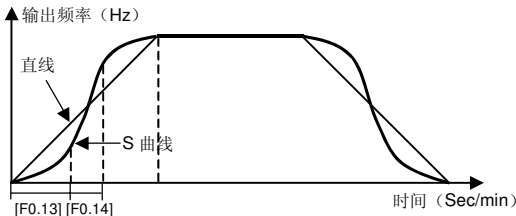
图 6-3 加 减 速 曲 线
