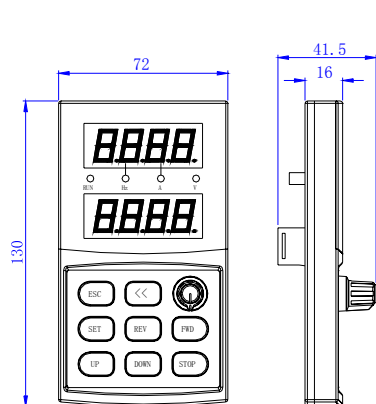
图-A 操作面板尺寸
