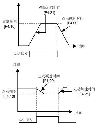
图 6-18 点动运行
