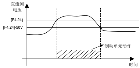
图 6-22 能耗制动
