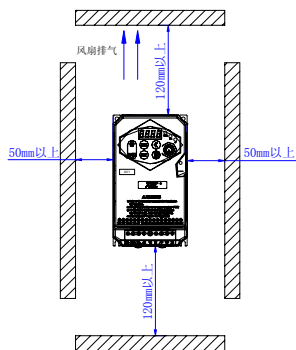
图 2-1-A 安装的间隔距离
