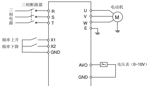
图 9-3 基本接线图
