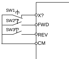
图 6-1 三线控制模式接线图
