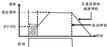
图 6-12 启动与停机频率输出曲线
