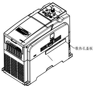
图 2-1-A 散热孔盖板的安装
