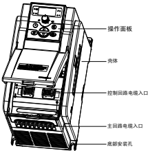
图 1-3 III类变频器外观及部件名称
