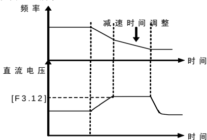
图 6-16 减速中的电压失速保护
