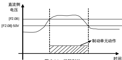
图 6-14 能耗制动
