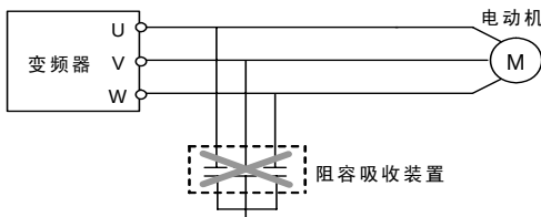
图 3-1 输出端禁止连接阻容吸收装置
