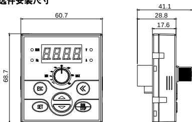
图 2-2-C 小键盘安装尺寸
