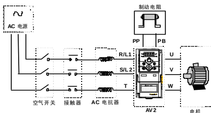
图 3-2 变频器的配线
