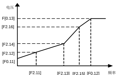
图 6-15 V/F 自定义曲线设定
