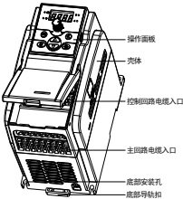
图 1-2 II类变频器外观及部件名称
