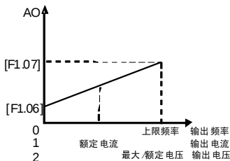
图 6-7 模拟输出端子的模拟输出内容
