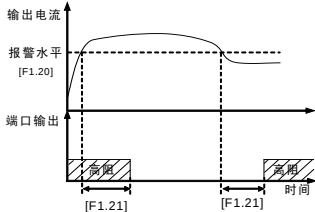
图 6-11 过载报警
