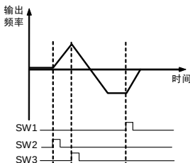
图 6-2 三线控制模式频率输出图
