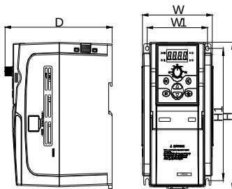
图 2-2-B 变频器安装尺寸 2
