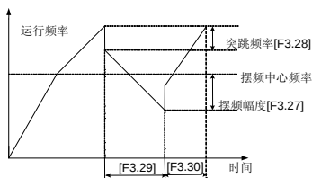
图 6-17 摆频运行过程
