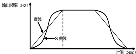
图 6-3 加减速曲线
