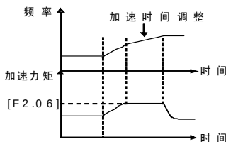
图 6-13 加速力矩与制动力矩示意图
