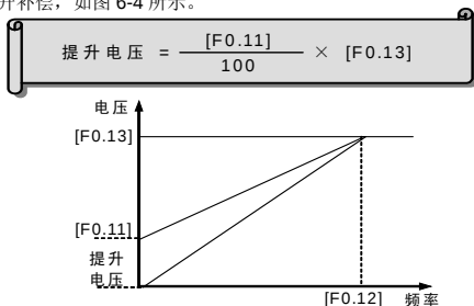
图 6-4 转矩提升示意图
