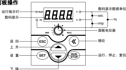
图 4-1 操作面板示意图
