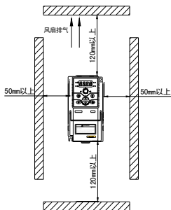
图 2-1-B 安装的间隔距离
