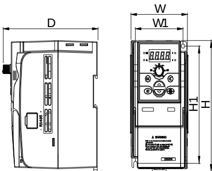
图 2-2-A 变频器安装尺寸 1
