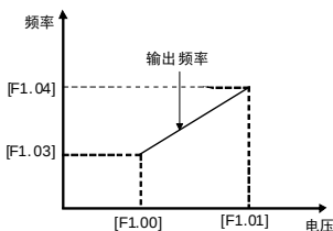
图 6-6 模拟输入量与设定频率对应关系图示
