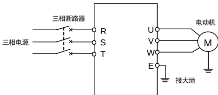
图 4-2 简单运行接线图
