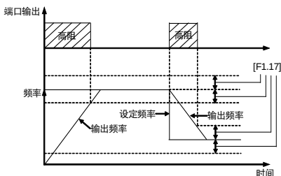
图 6-9 频率到达信号
