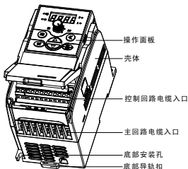
图 1-1 I 类变频器外观及部件名称
