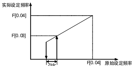
图 6-5 下限频率作用示意图
