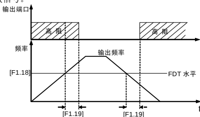
图 6-10 频率水平检测信号 (FDT)
