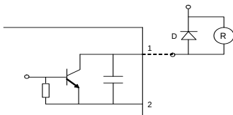
图 6-8 OC 输出端子的内部线路
