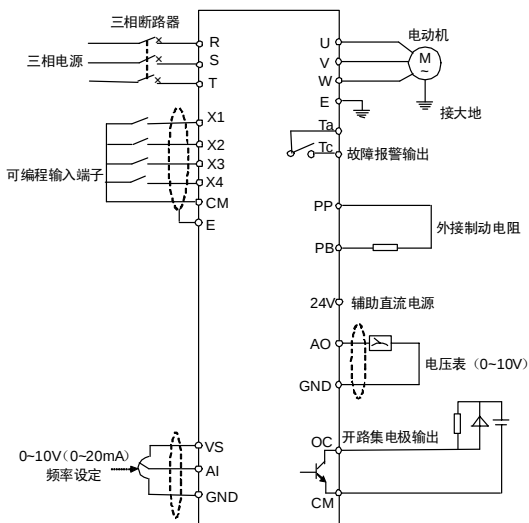
图 3-3 变频器的基本配线
